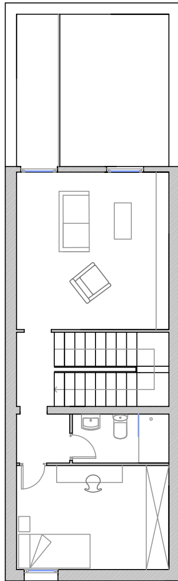
Planta primera
